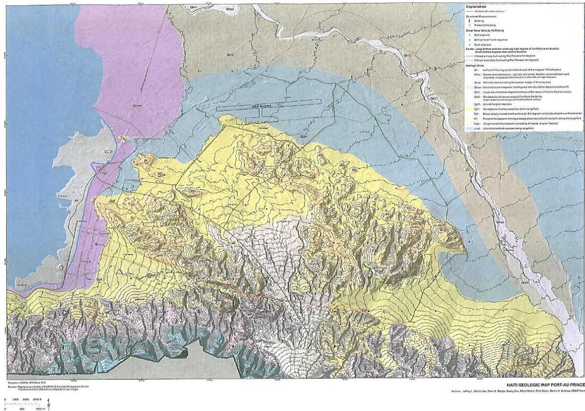
Carte géologique préliminaire de Port-au-Prince, d'après Bachhuber et al. (2010)
